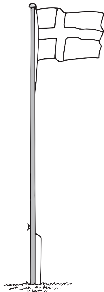
Træflagstænger: længde, diameter og vægt.
